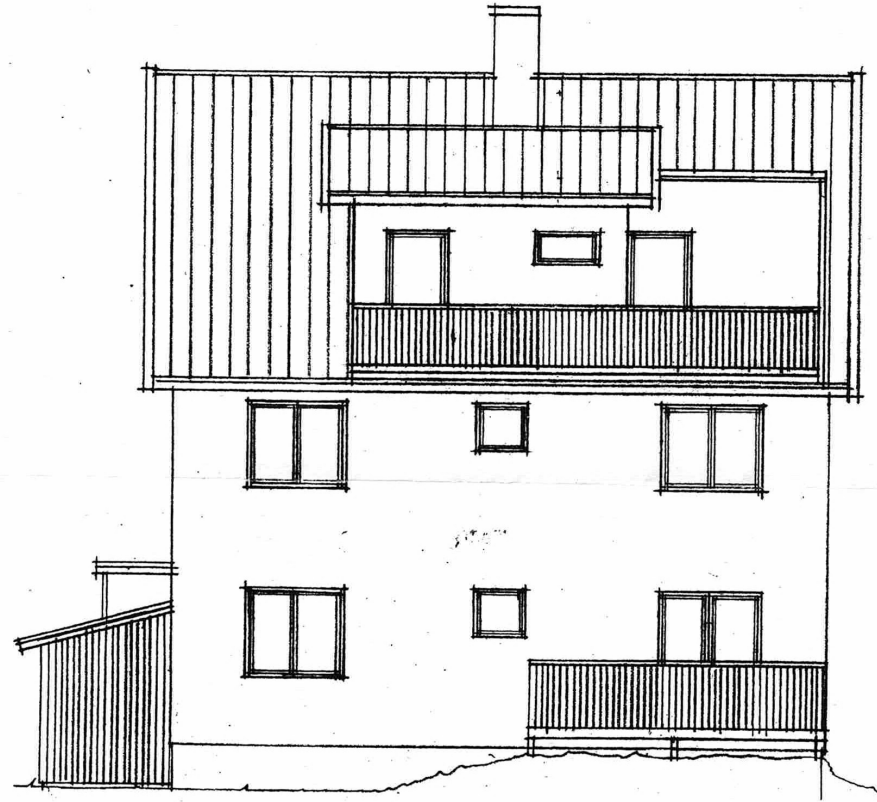
Fasad mot väster
