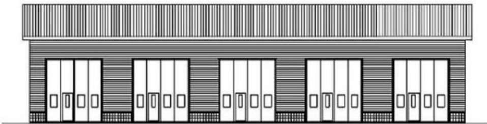
Enkel access till lagerdelen genom den 4 meter breda och 4,5 meter höga industriporten.
